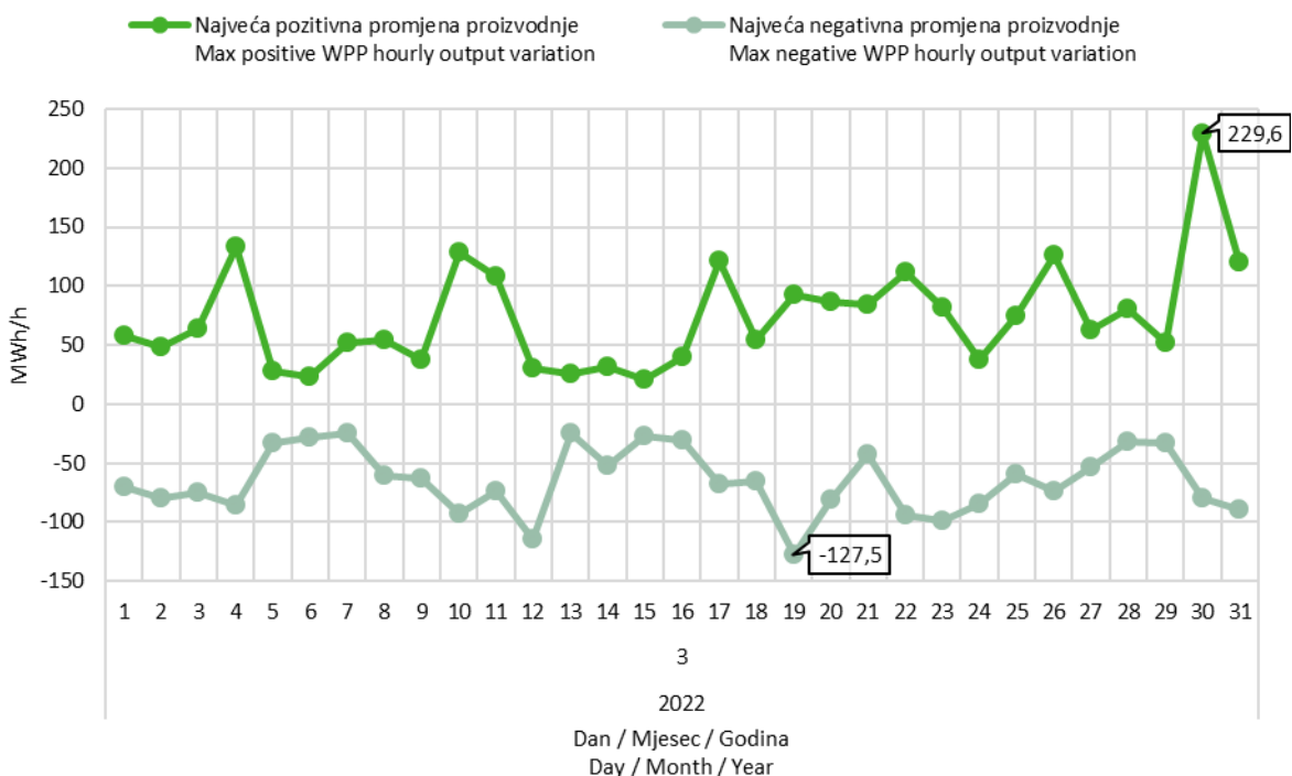
Slika 9 Maksimalna pozitivna i maksimalna negativna promjena satne proizvodnje VE u ožujku 2022. godine
