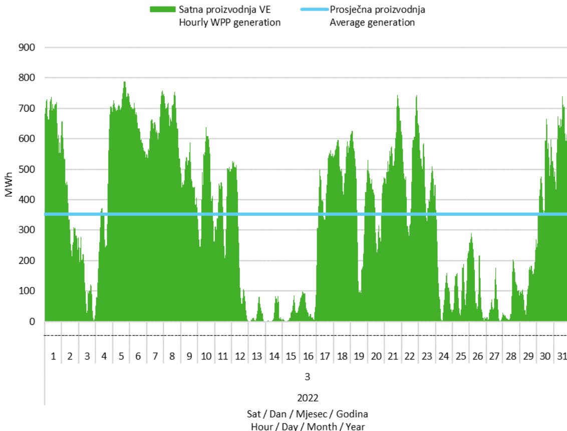
Slika 2 Satna proizvodnja svih vjetroelektrana u ožujku 2022. godine
