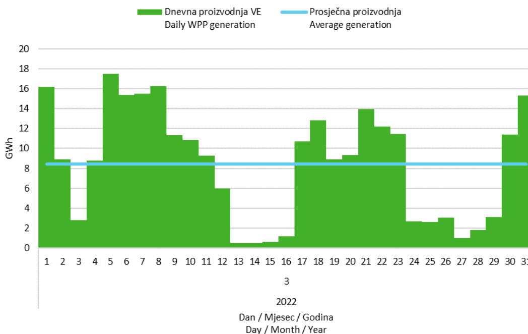
Slika 5 Dnevna proizvodnja svih vjetroelektrana u ožujku 2022. godine
