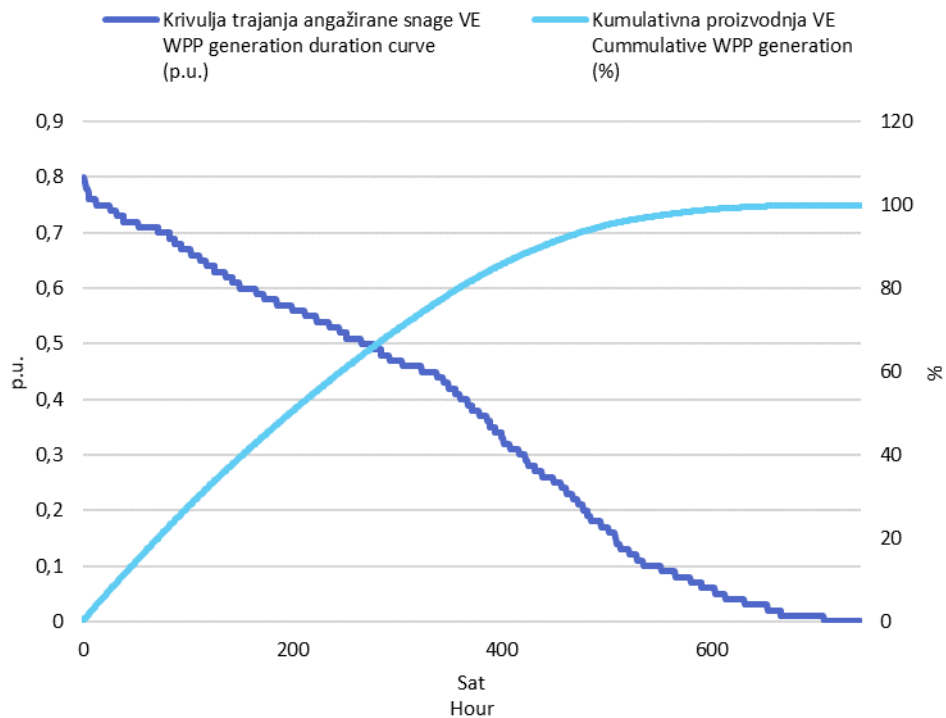
Slika 3 Krivulja trajanja angažirane snage svih VE i kumulativna proizvodnja VE u ožujku 2022. godine u jediničnim vrijednostima
