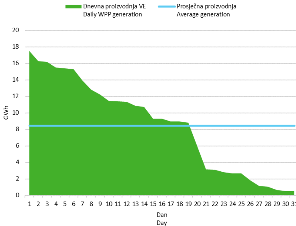
Slika 6 Krivulja trajanja dnevne proizvodnje vjetroelektrana u ožujku 2022. godine
