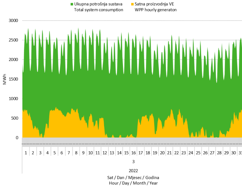
Slika 7 Usporedba satnog dijagrama opterećenja sustava i proizvodnje vjetroelektrana u ožujku 2022. godine
