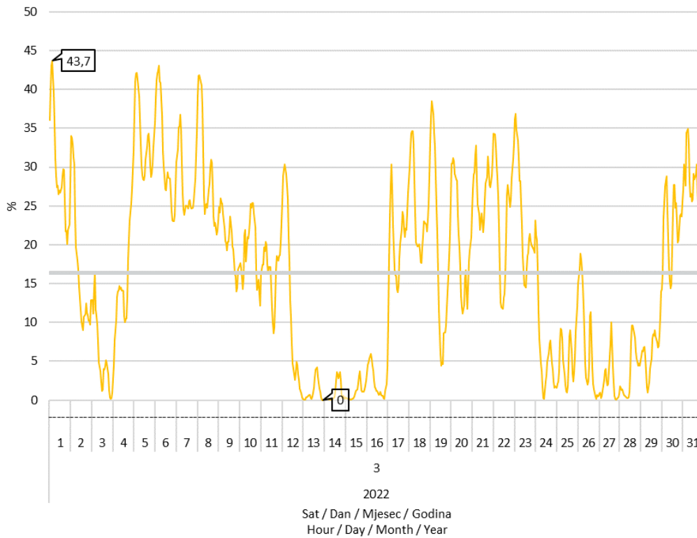
Slika 8 Udio proizvodnje vjetroelektrana u pokrivanju satnog opterećenja elektroenergetskog sustava u ožujku 2022. godine
