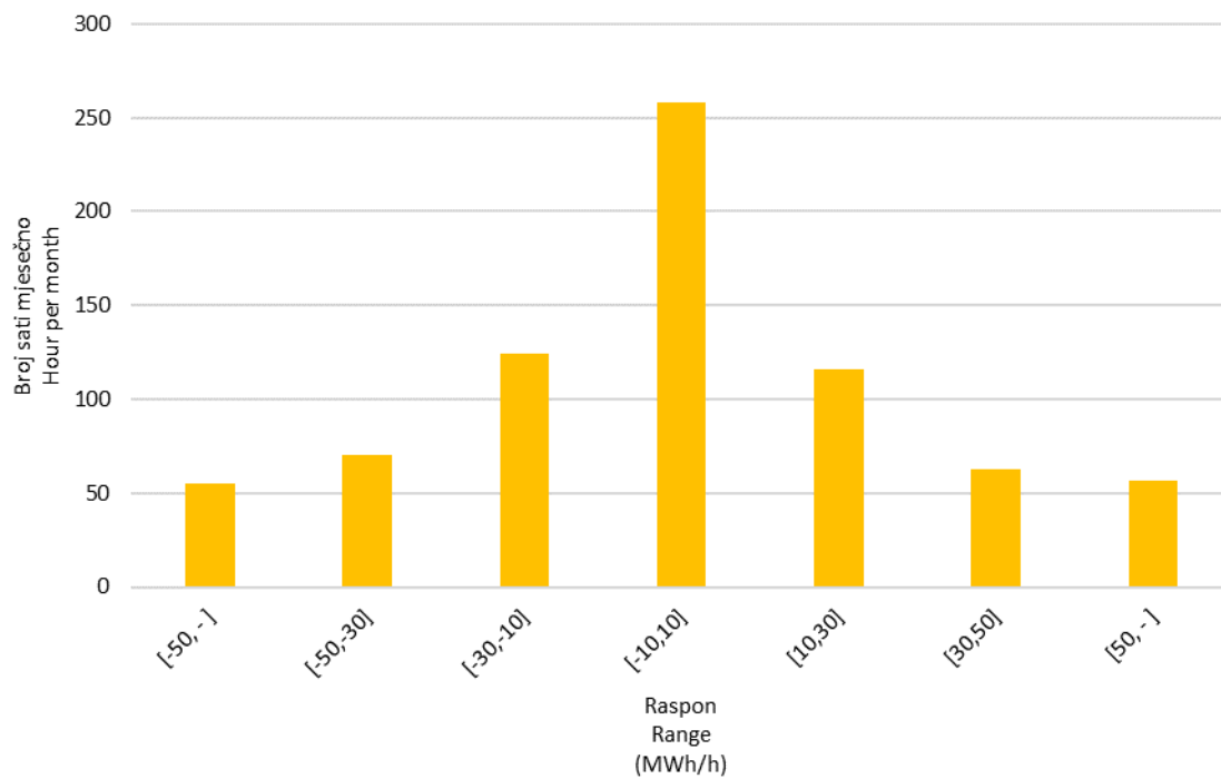
Slika 10 Statistička raspodjela satnih promjena proizvodnje VE u ožujku 2022. godine
